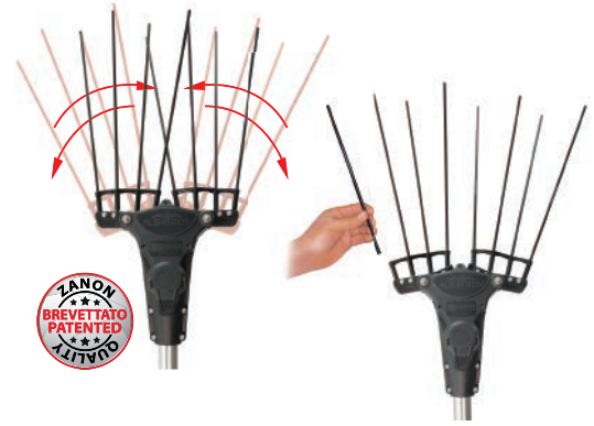
Tiges en carbone de remplacement facile et rapide Easy and quick replacement carbon rods Einfacher und schneller Austausch von Karbonstäbchen
